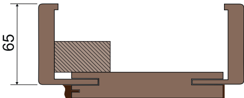
protipožární obložková zárubeň profil č. 1
