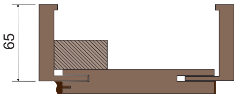
protipožární obložková zárubeň profil č. 6
