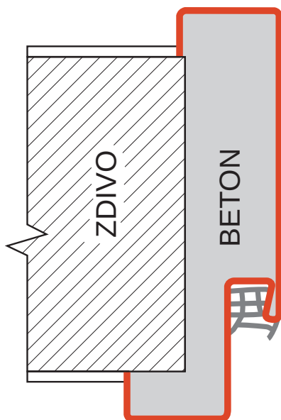
Bezpečnostní a protipožární ocelová zárubeň s těsněním pro klasické zdění
