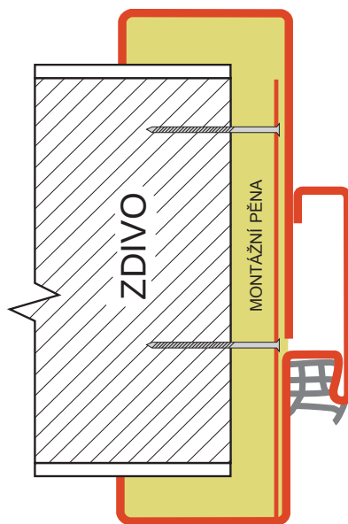
Bezpečnostní a protipožární ocelová zárubeň s těsněním pro dodatečnou montáž
