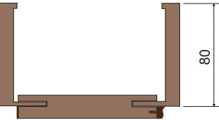
profil zárubně č. 3
