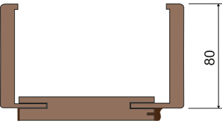
profil zárubně č. 2
